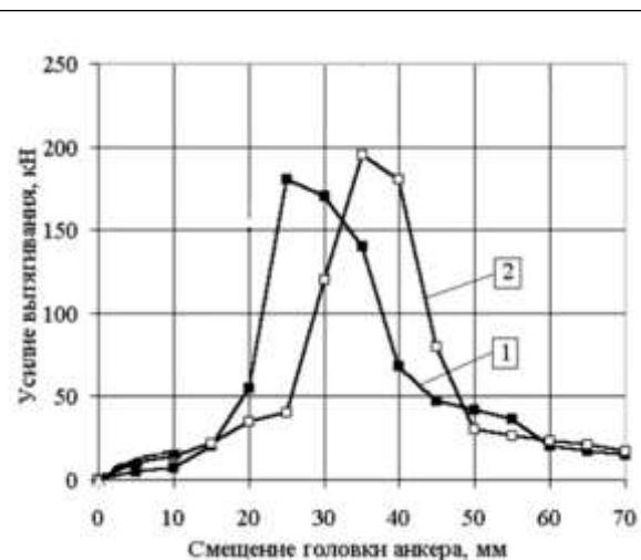
1 – нижняя граница смещений анкеров; 2 – верхняя граница смещений анкеров
